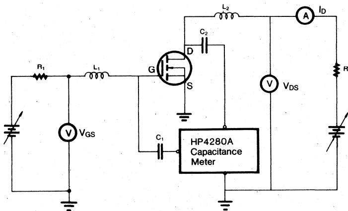
Fig. 6. C_{rss} Test Circuit
